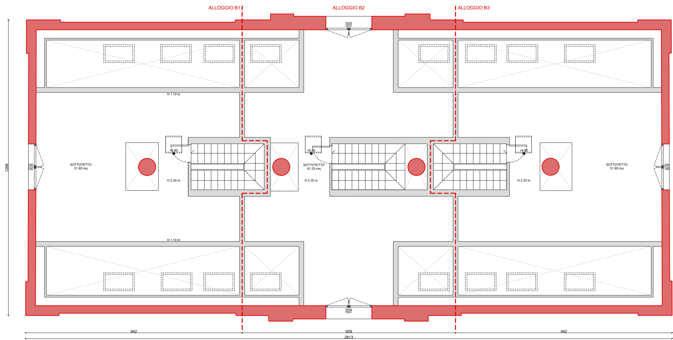
PLANIMETRIA PIANO SECONDO
