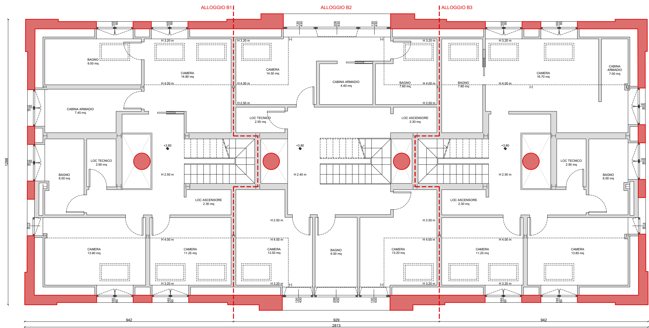
PLANIMETRIA PIANO PRIMO
